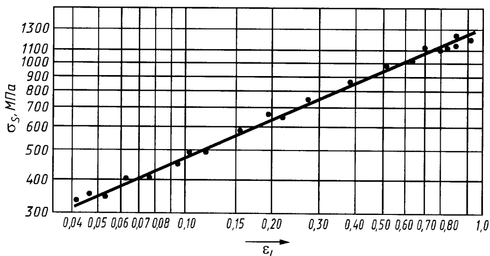
Рисунок 10 — Экспериментальная кривая упрочнения в логарифмических координатах
