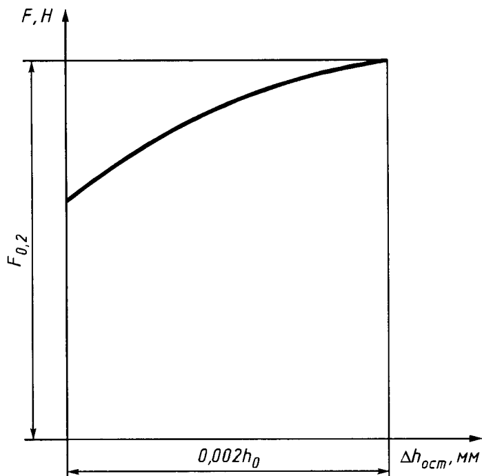
Рисунок 7 — Диаграмма испытаний для определения условного предела текучести при сжатии
