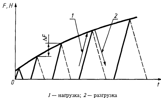
Рисунок 11 — Проведение испытаний при ступенчатом увеличении нагрузки
