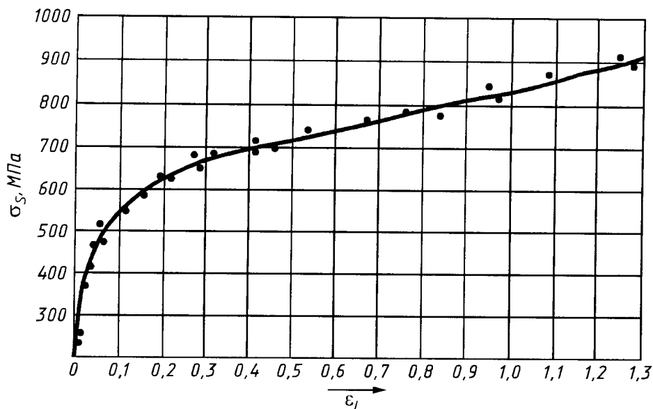
Рисунок 9 — Экспериментальная кривая упрочнения в координатах \sigma_s - \epsilon_l
