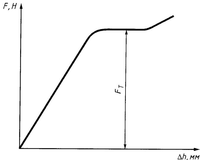
Рисунок 6 — Определение нагрузки F_T , соответствующей пределу текучести при сжатии
